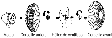
Moteur Corbeille arrière Hélice de ventilation Corbeille avant
